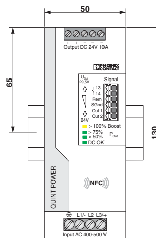
Disegno quotato
