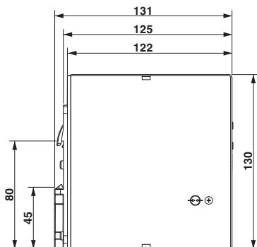
Disegno quotato
